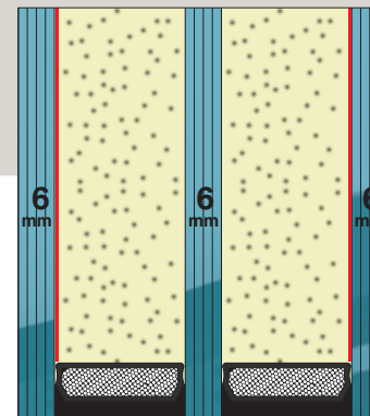
Ug-Wert 0,5\text{ W/m}^2\text{K}
